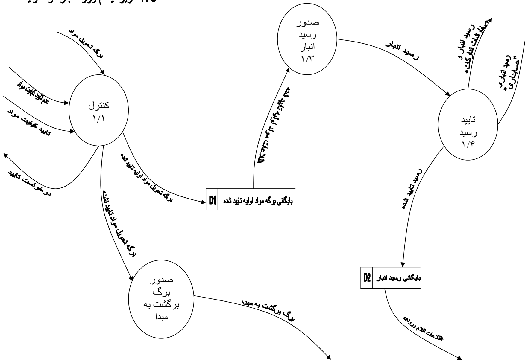
شکل 17- زیرسیستم ورود انبار مواد اولیه
